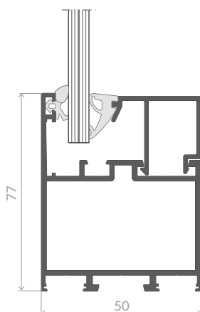
Przekrój przez futrynę stałą
