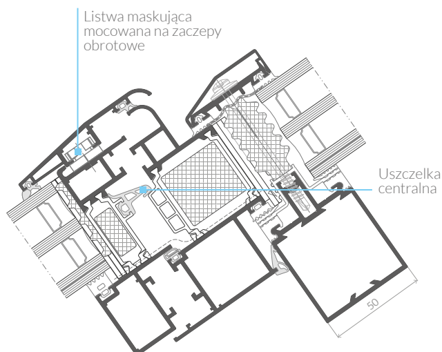
Przekroj przez okno połaciowe w fasadzie
