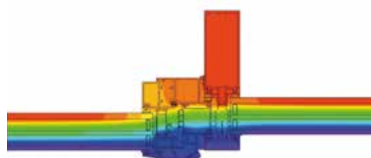
Rozkład temperatur
