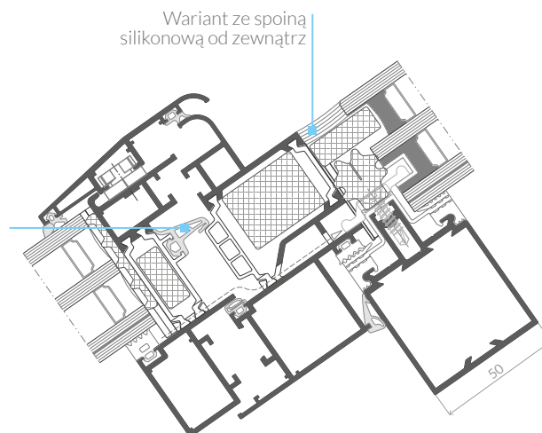
Przekroj przez okno połaciowe w fasadzie silikonowej
