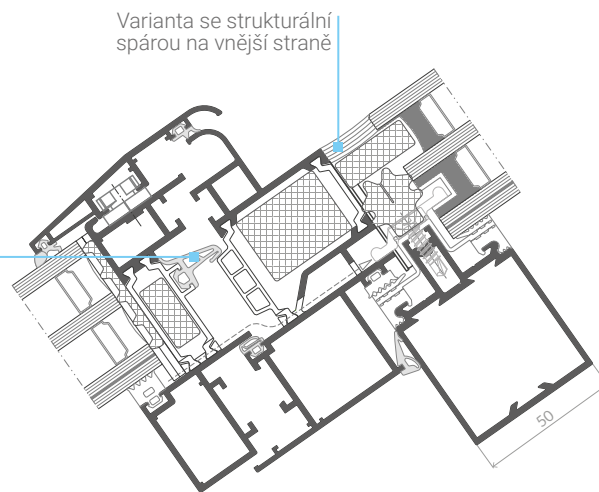
Řez střešního okna ve strukturální fasádě
