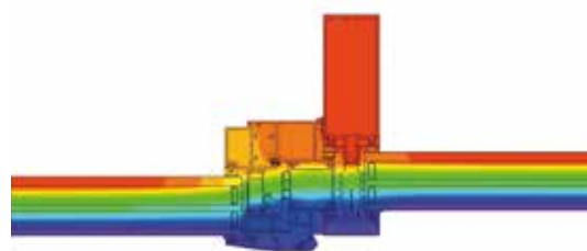
Rozložení teplot
