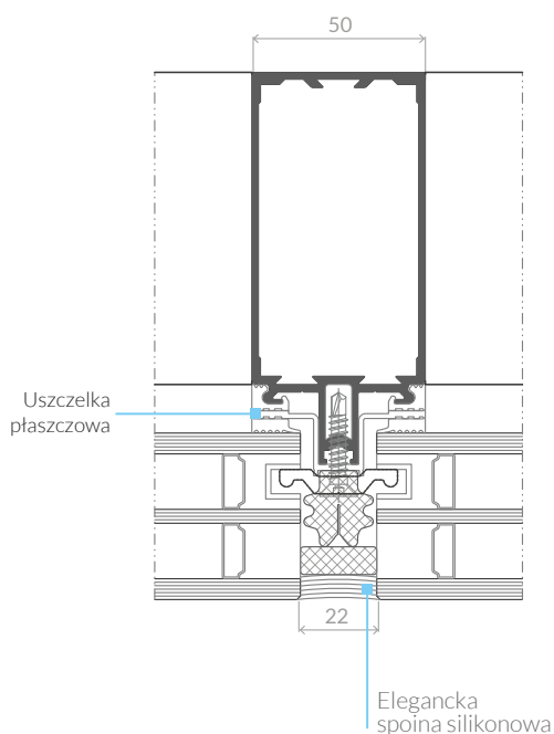
Przekrój przez słup
