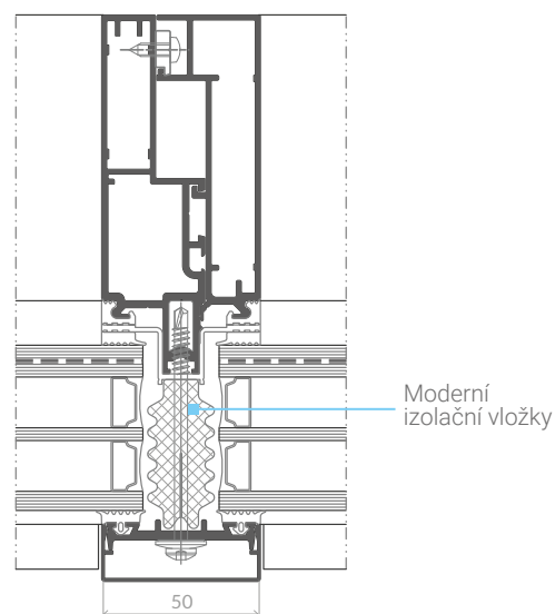
Řez sloupku – pevný díl
