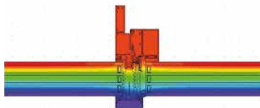
Rozložení teplot
