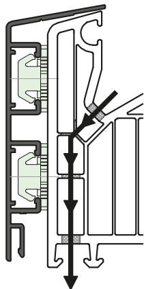
Rys. 2. – Odprowadzenie wody od dołu
