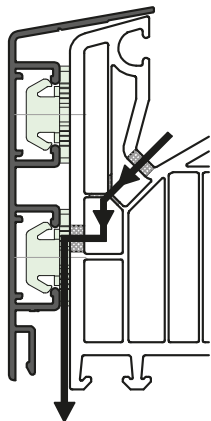
Rys. 1. – Odprowadzenie wody od czoła
