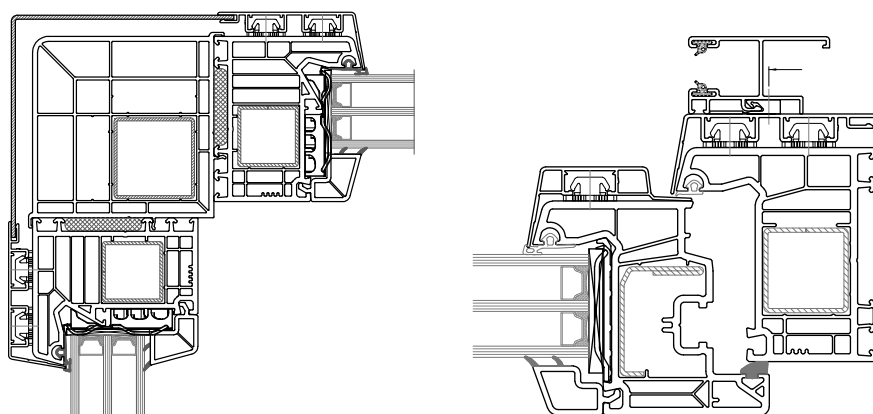
Profil kątowy
