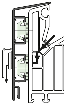
Rys. 3. – Odprowadzenie wody od czoła + zaślepka alu
